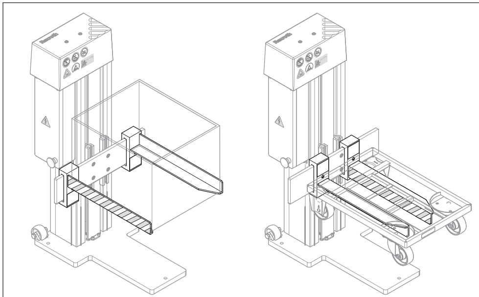
Fig. 4: Bruksområde gaffel for kasseløfter, elektrisk
