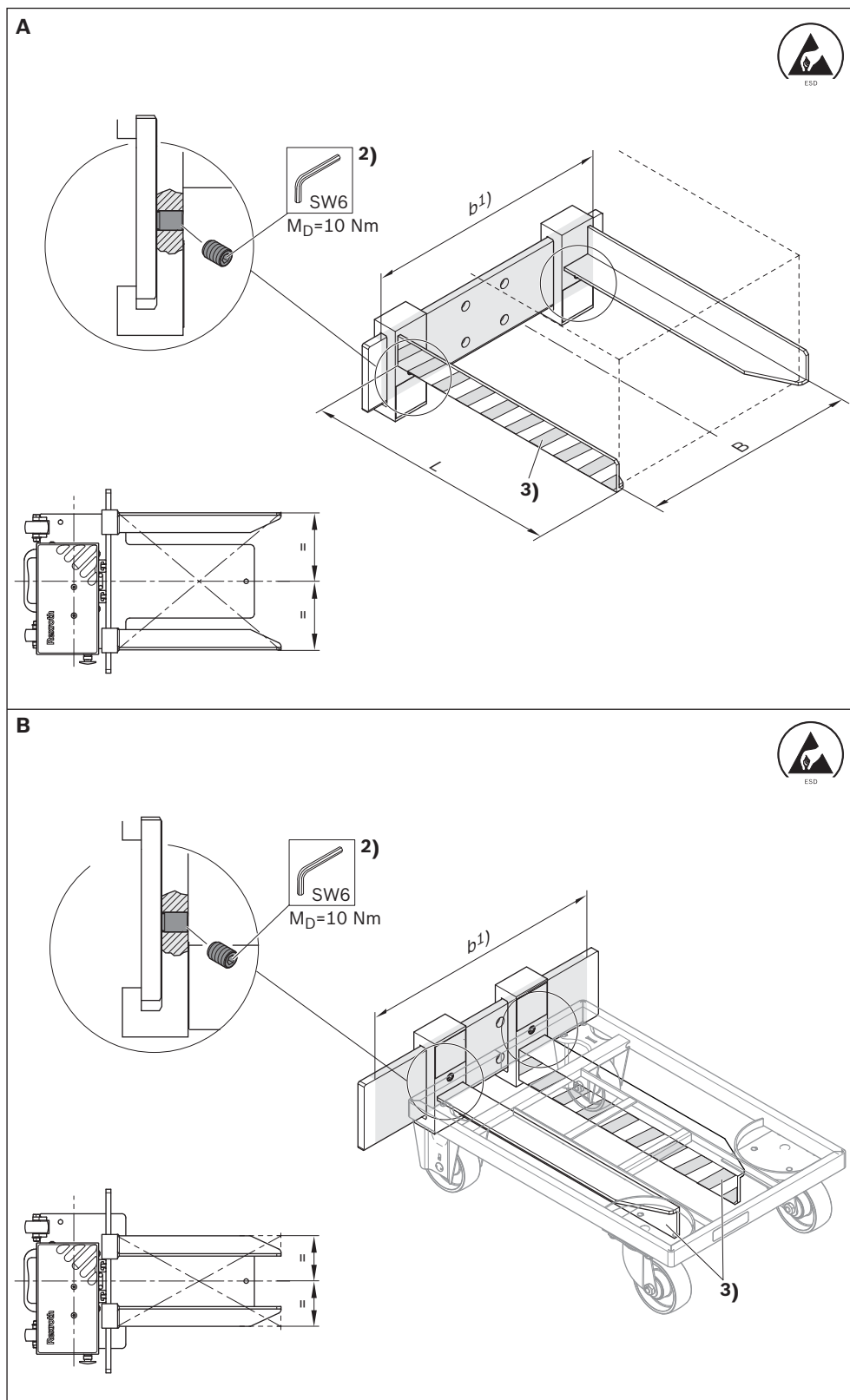
Fig. 10: Justere gaflene
