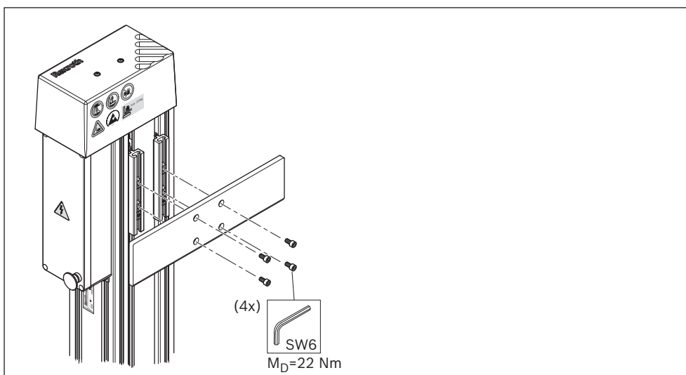
Fig. 11: Tiltrekkingsmoment på skruene som holder monteringsplaten
