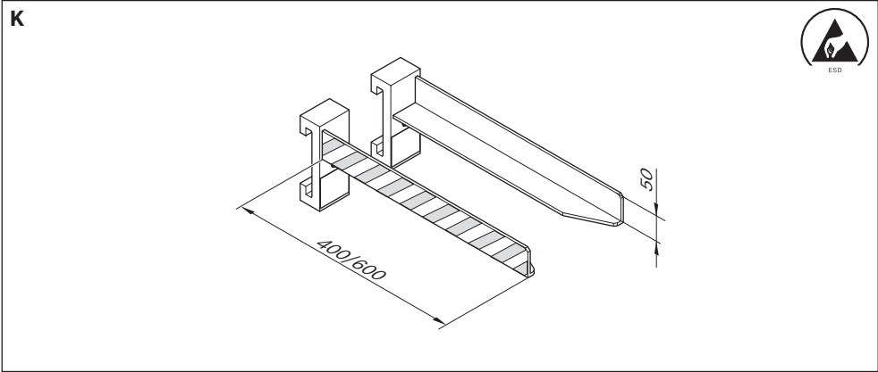
Fig. 5: Produktbeskrivelse kasseløfter, elektrisk
