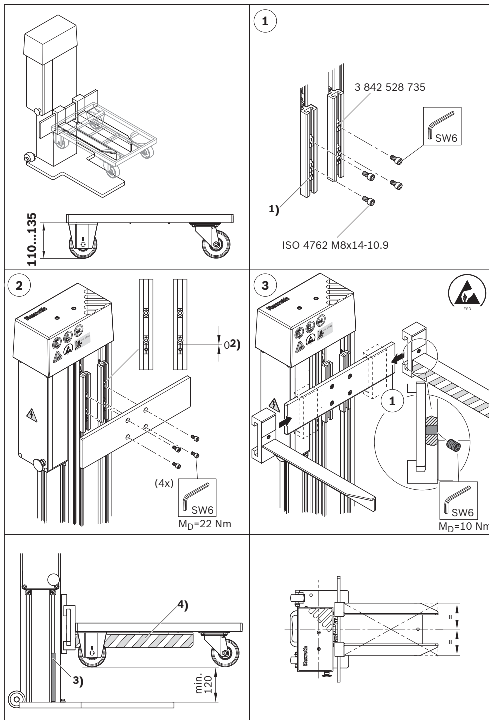
Fig. 8: Montering monteringsplate, gafler for hjultraller med en bakkeklaring på 135 mm
