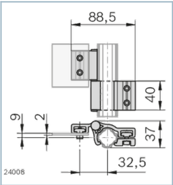
Hinge D28L/-
