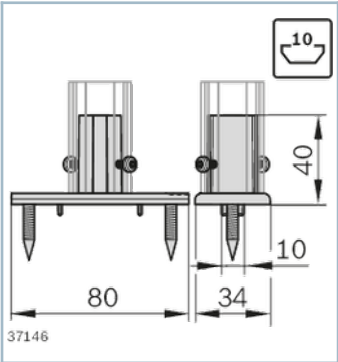
D28L base plate
